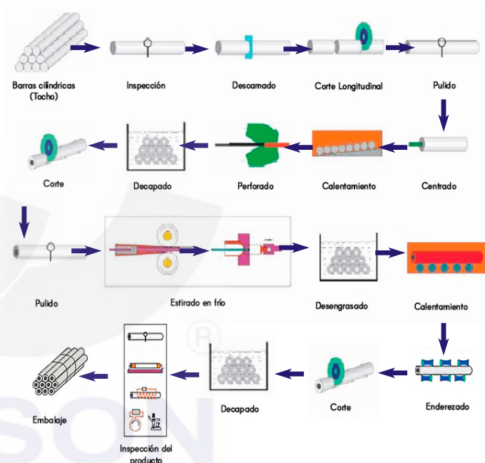
Figura 1. Proceso productivo, tubos sin costura
